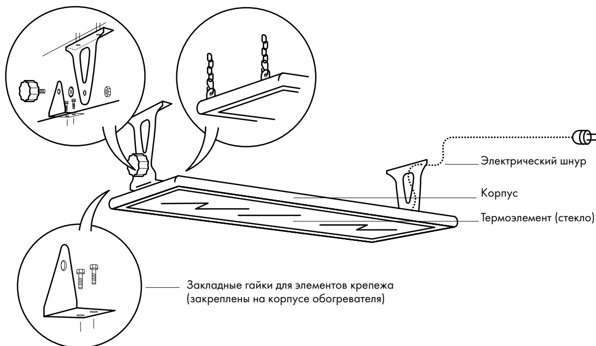
Схема 3. Обогреватель ThermoUp Top 700/1100/1500
